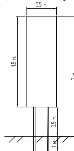
Макет двусторонней отдельностоящей рекламной конструкции
