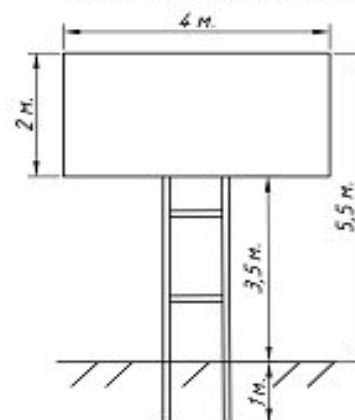
Макет двусторонней отдельностоящей рекламной конструкции
